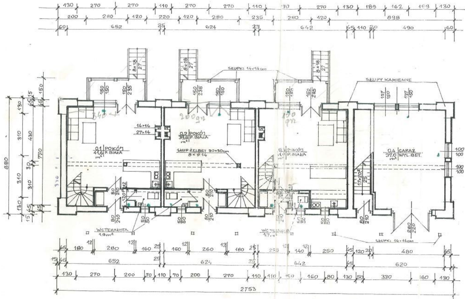
Powozownia rzut parteru
