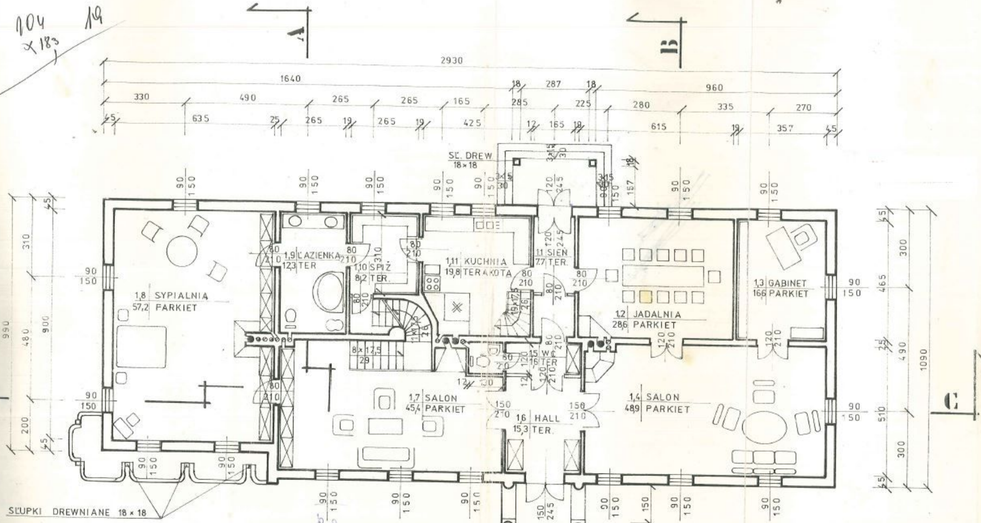
Dwór rzut parteru
